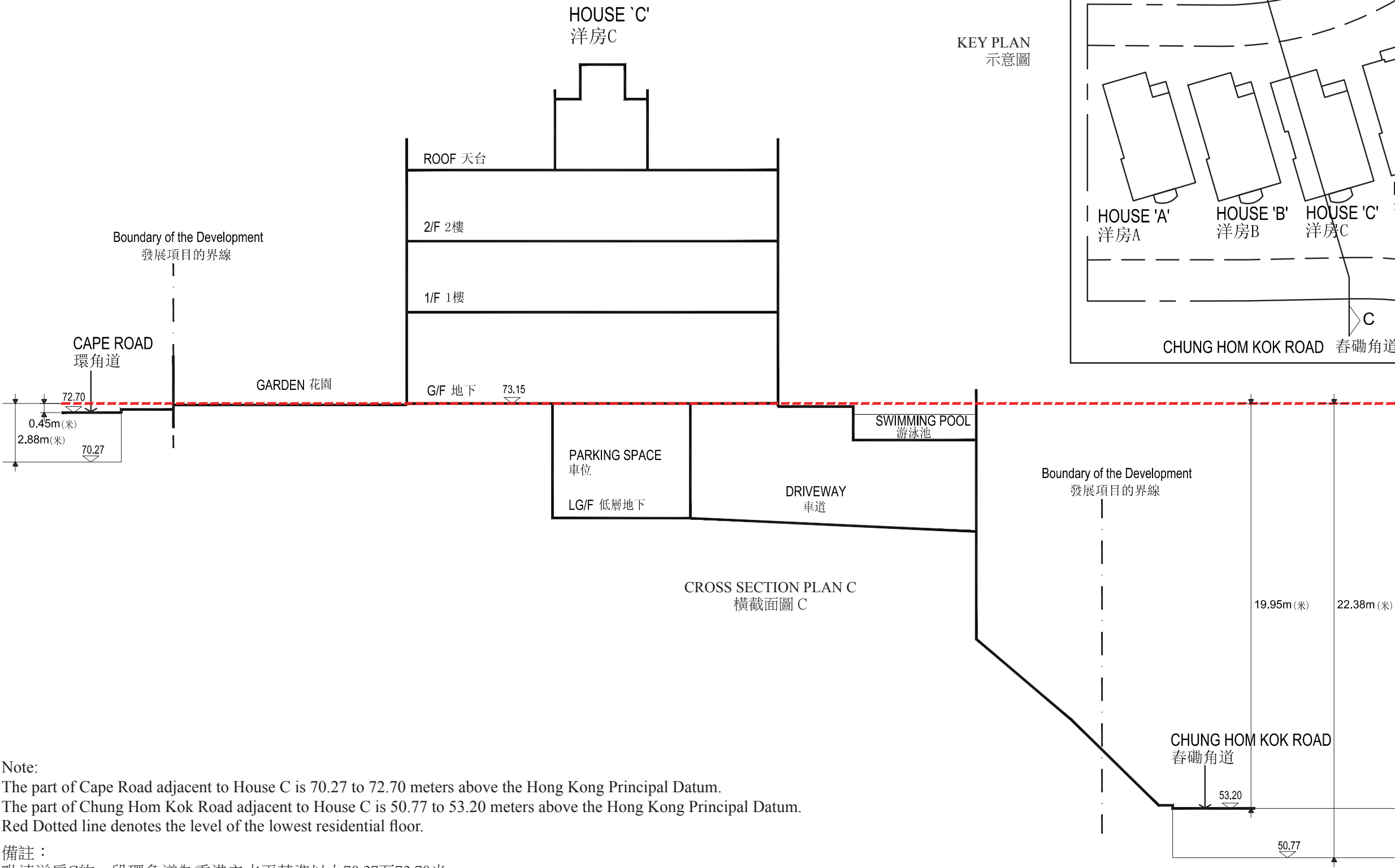
House C - Cross Section Plan 洋房 C - 橫截面圖
